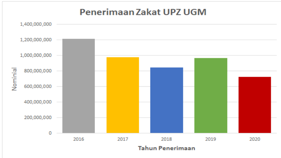
Gambar 1.1. Histogram Penerimaan Zakat UPZ UGM
